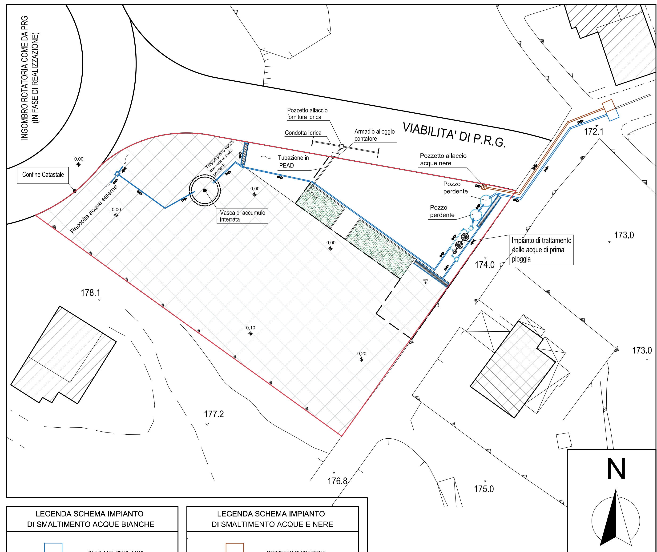
PLANIMETRIA GENERALE CON INDICAZIONE SCHEMA IMPIANTO DI SMALTIMENTO ACQUE BIANCHE E NERE ED ALLACCIO FORNITURA IDRICA Scala 1:400
